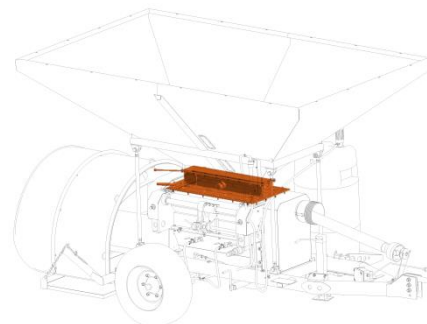
07 GRAIN DOSING
